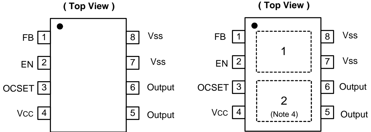
(1) SOP-8L
